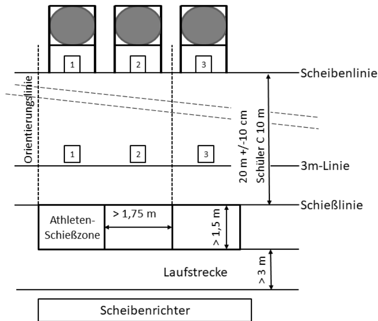
Abb. 9: Aufbau des Schießbereichs
